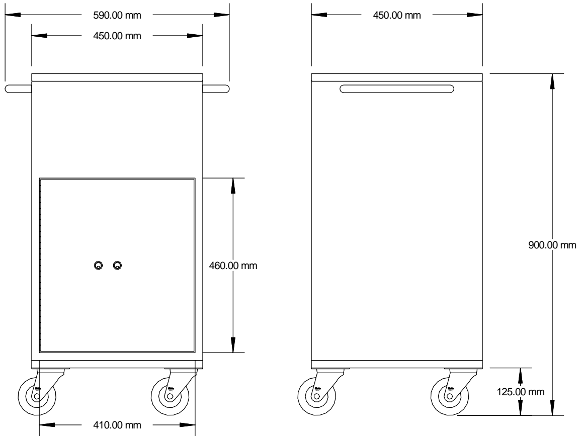
Sealbag trolley, 450 x 450
